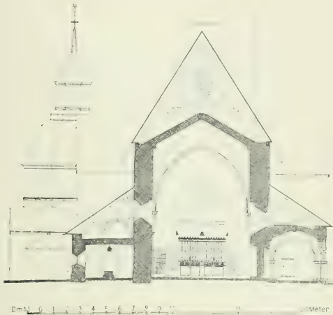
Fig. 26. Tvärsektion genom korets västra valv samt »Magnus Nilssons» gravkor och »Norra förhallen». Efter uppmätning av S. Curman o. A. Roland 1907, kompletterad av H. Sundberg 1927.
